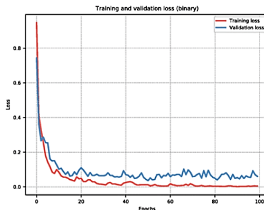
نمودار ۹: فرآیند کاهش خطا برای مرحله آموزش در معماری منتخب CNN
